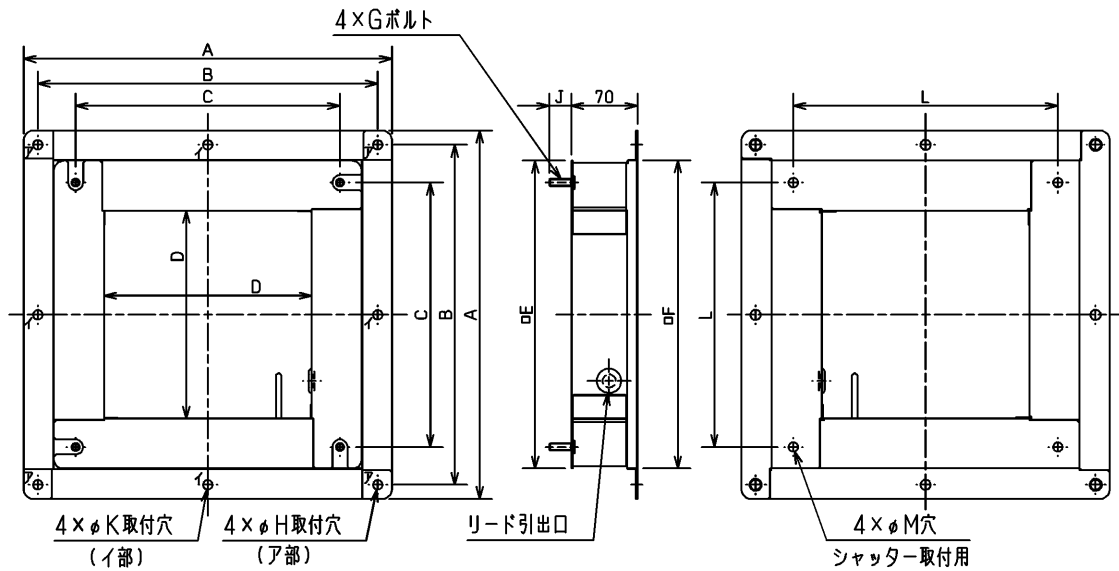
変化寸法表
