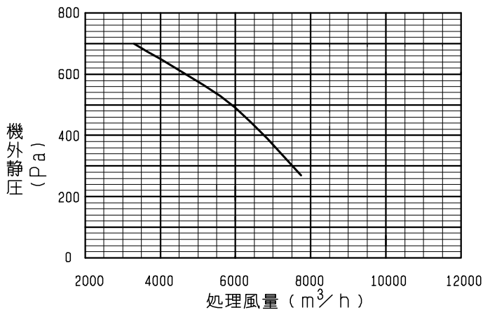
LP-750X 3 , X 4
