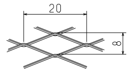
防鳥網 詳細
