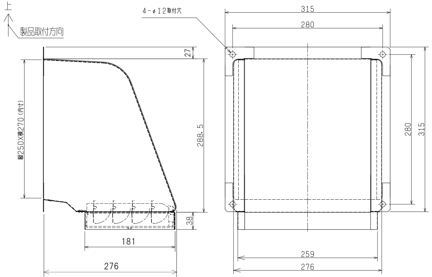
防鳥網 詳細
