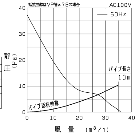
P-Q特性図
