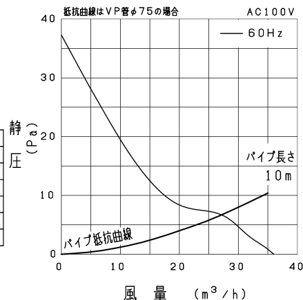
P-Q特性図
