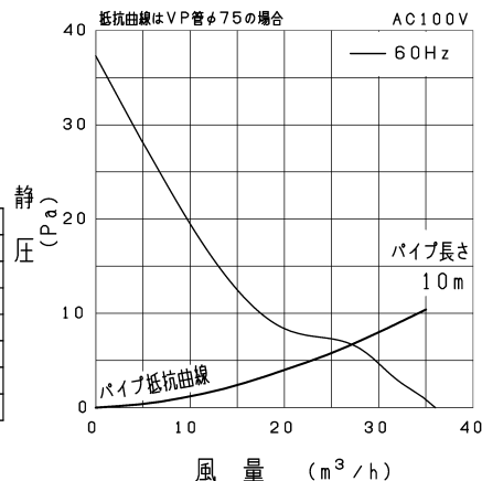
P-Q特性図
