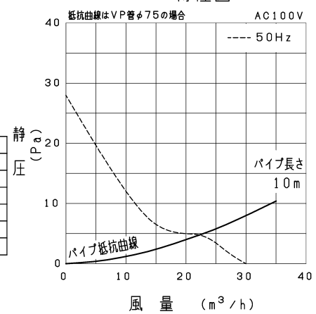
P-Q特性図
