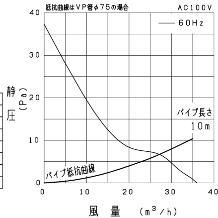
P-Q特性図
