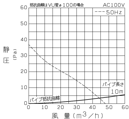
P-Q特性図
