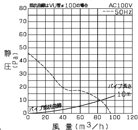
P-Q特性図
