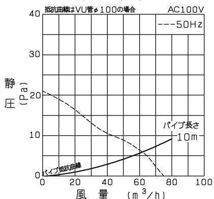
P-Q特性図
