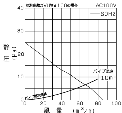
P-Q特性図
