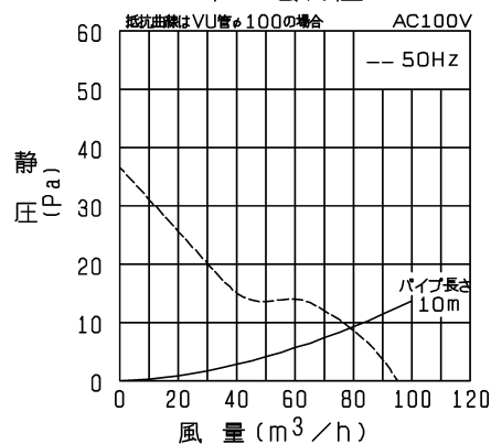
P-Q特性図
