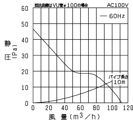
P-Q特性図
