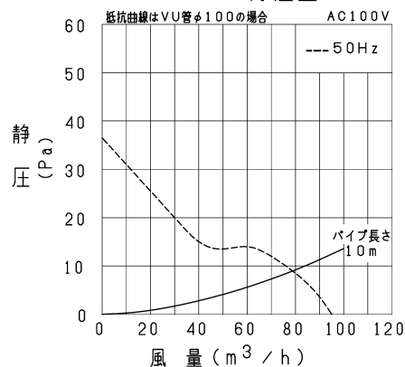
P-Q特性図
