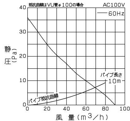
P-Q特性図
