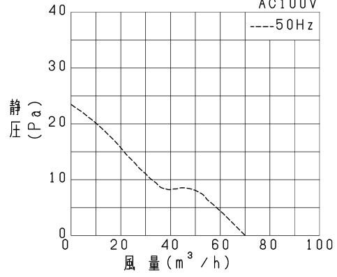
P-Q特性図
