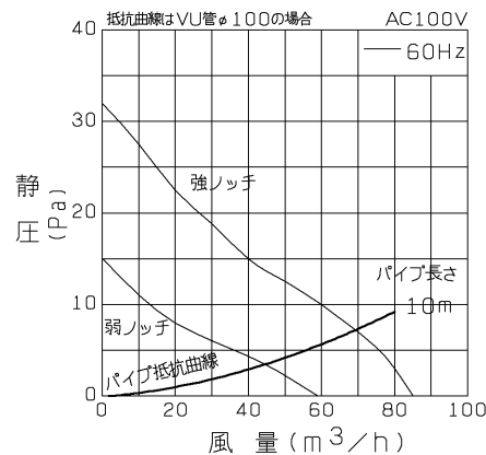
P-Q特性図
