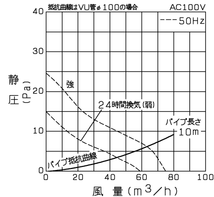
P-Q特性図
