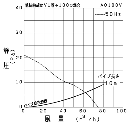
P-Q特性図
