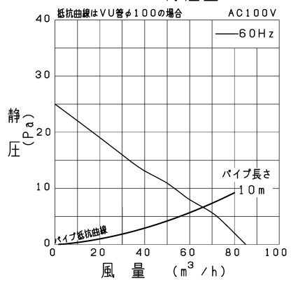
P-Q特性図
