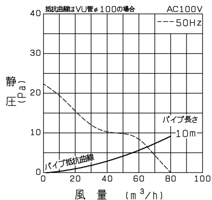
P-Q特性図
