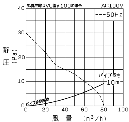
■ P-Q特性図
