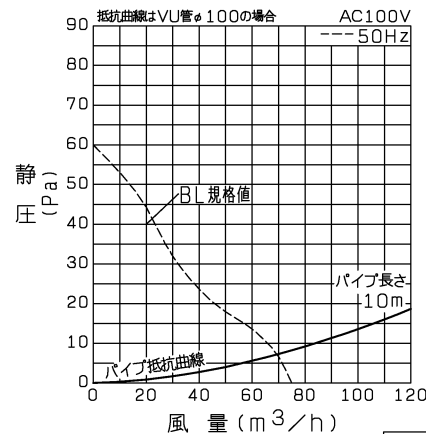
P-Q特性図
