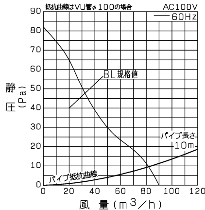
P-Q特性図
