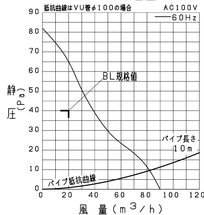
P-Q特性図
