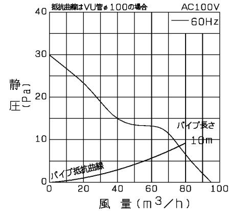
P-Q特性図
