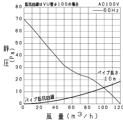
P-Q特性図
