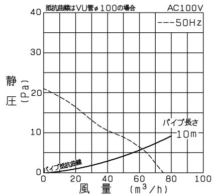
■ P-Q特性図
