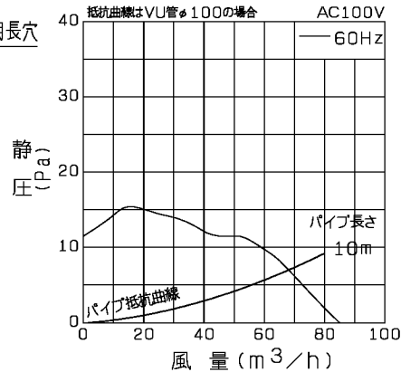
P-Q特性図
