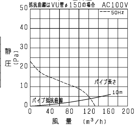
P-Q特性図
