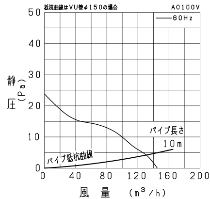
P-Q特性図
