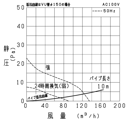
P-Q特性図
