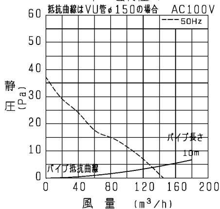
P-Q特性図
