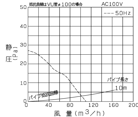
P-Q特性図
