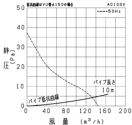
P-Q特性図
