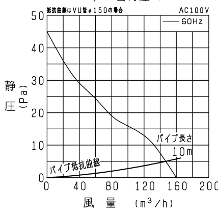
P-Q特性図
