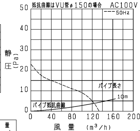
P-Q特性図
