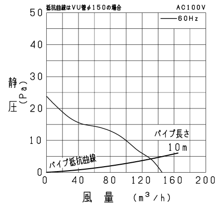
P-Q特性図
