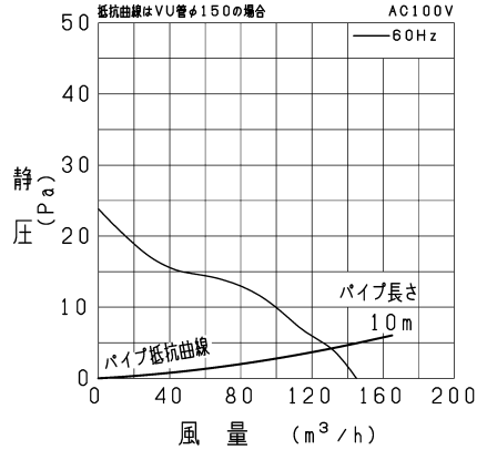
P-Q特性図
