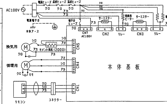
■ 結線図 破線部の結線はお客様にて施工してください。
