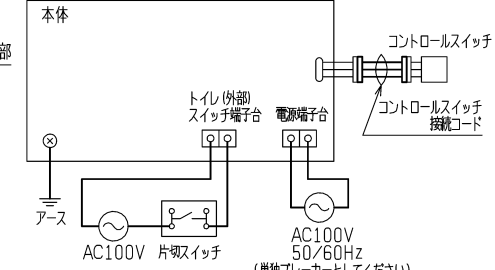
■ 結線図
