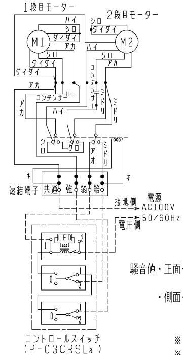
■ P-03CRSL 3 使用の運転回路 破線部分の結線はお客様にて施工してください。
