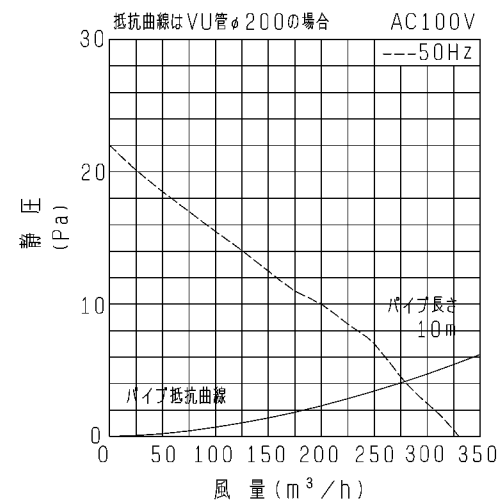
P-Q特性図
