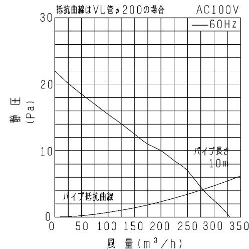
P-Q特性図
