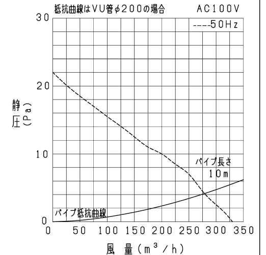
P-Q特性図
