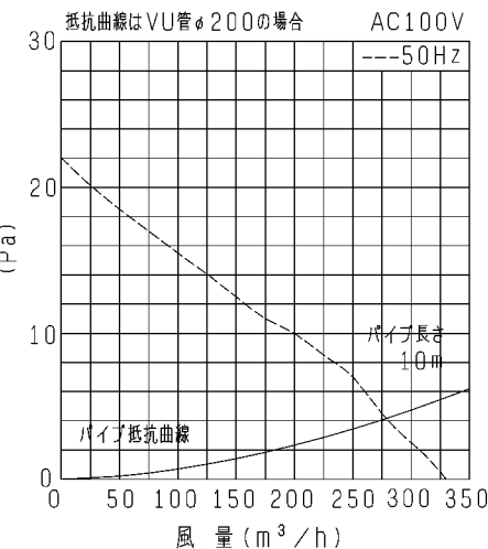
P-Q特性図
