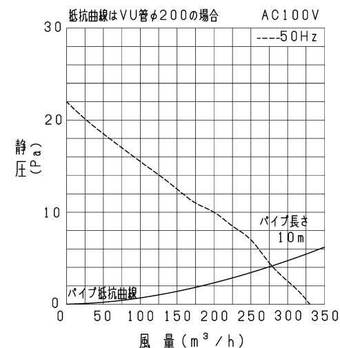
P-Q特性図
