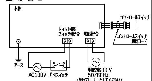
■ 結線図
