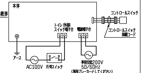
■ 結線図
